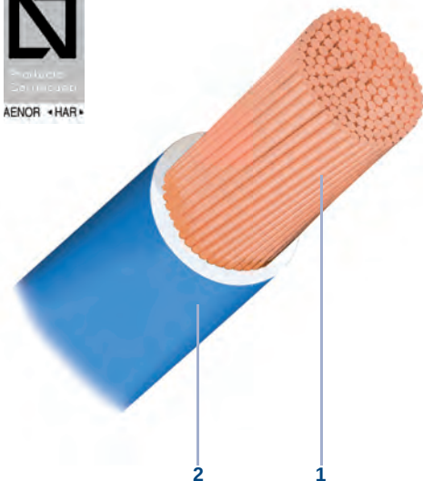
Simulação Cabo H07Z1-K(AS) type 2 1x1.5 mm 2
