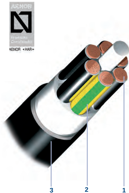
Simulação Cabo ES05VV-F 6 G1 mm 2
