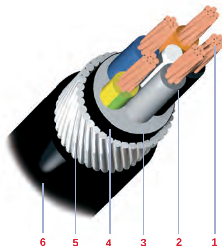
Simulação Cabo RVMV 0,6/1 kV 5G10 mm 2
