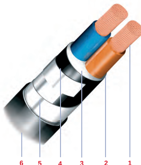
Simulação Cabo RVFEV-K 0,6/1kV 2 x 10 mm 2 .
