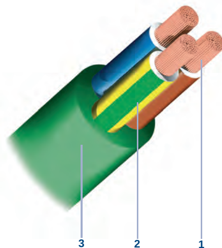
Simulação Cabo H05Z1Z1-F 3G1.5 mm²
