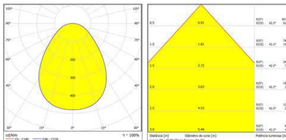
DL SLIM ALU D175 V 16W MS 830 WT
