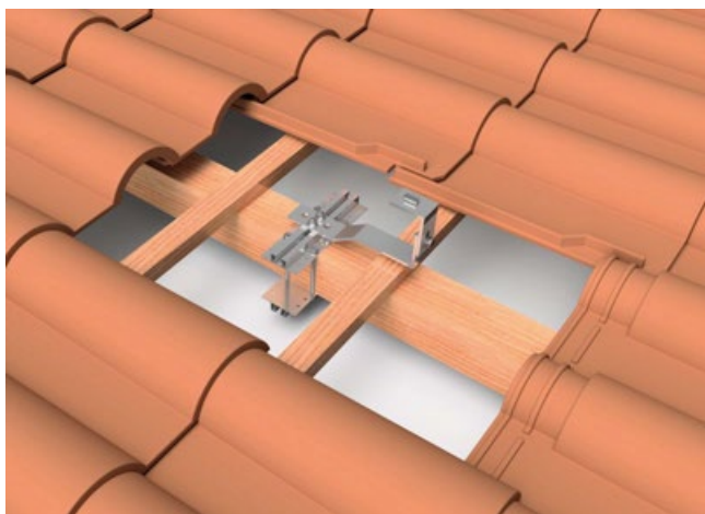
02.2V com acessório abraçadeira - Posição 2
