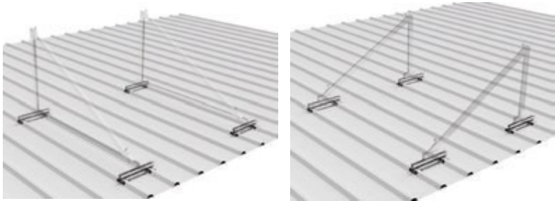
Para distâncias entre canelado ≤ 300 mm (triângulos não incluídos)
