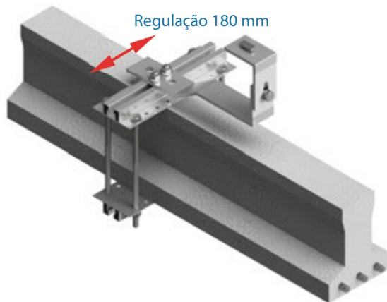
02.2V com acessório abraçadeira - Posição 1
