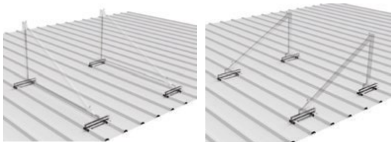
Para distâncias entre canelado ≤ 1000 mm (triângulos não incluídos)
