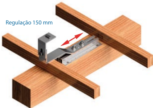
02.2V com acessório aparafusado
