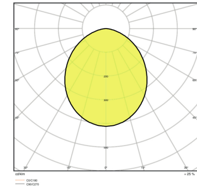
FL PFM 80 W 6500 K SYM 100 BK
