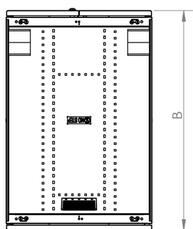
Vista superior (600 mm de largura)
