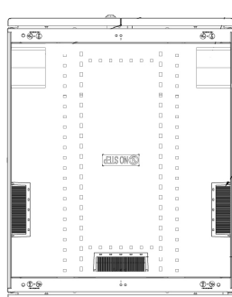
Vista superior (800 mm de largura)
